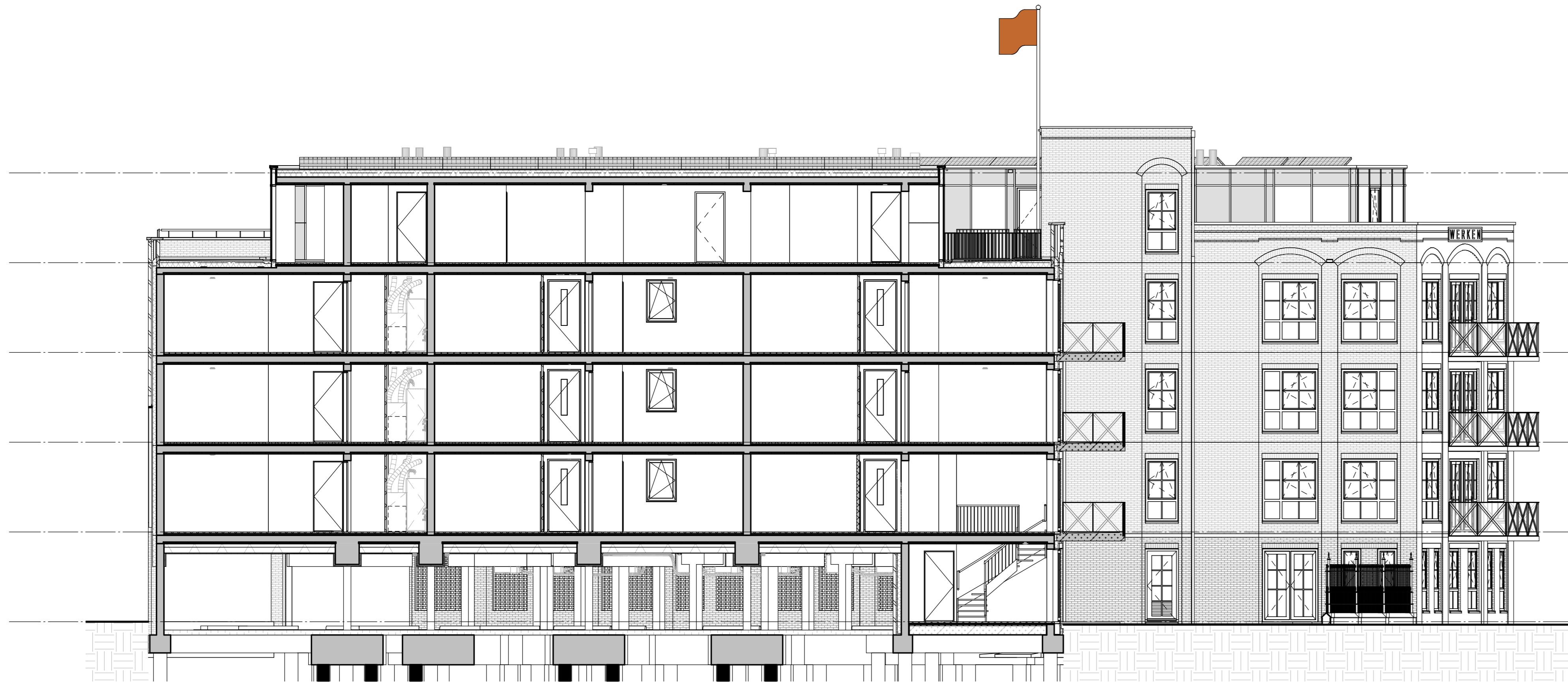
langsdoorsnede A-A Wittoucksingel
