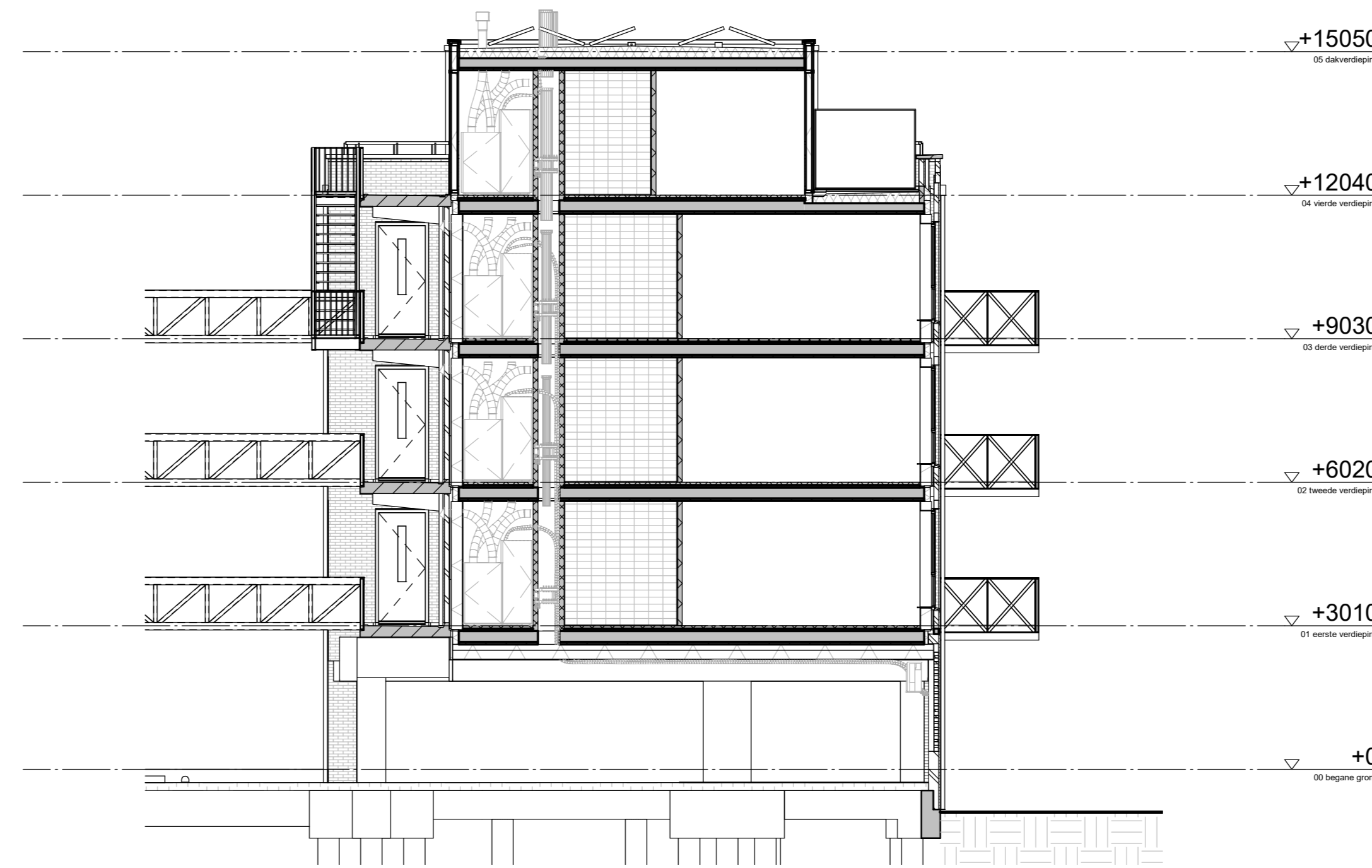
dwarsdoorsnede C*-C* Oude Vissershaven
