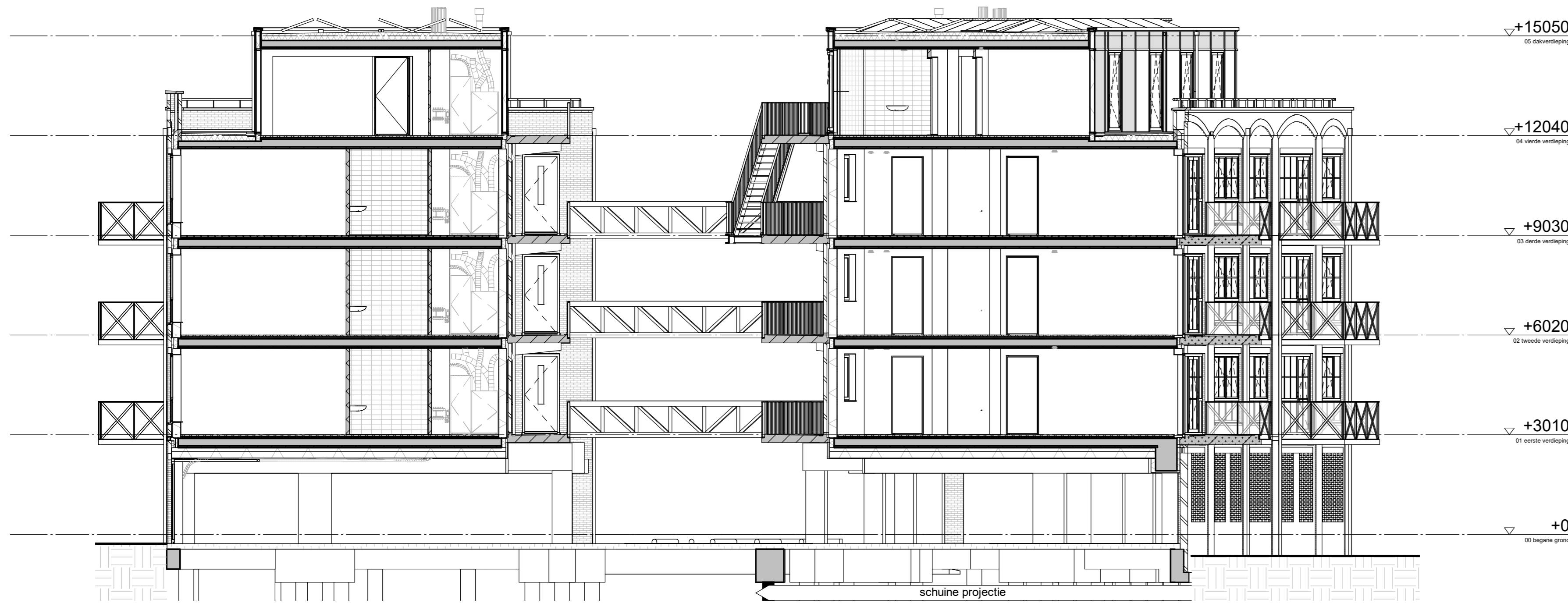
dwarsdoorsnede C-C Wittoucksingel
