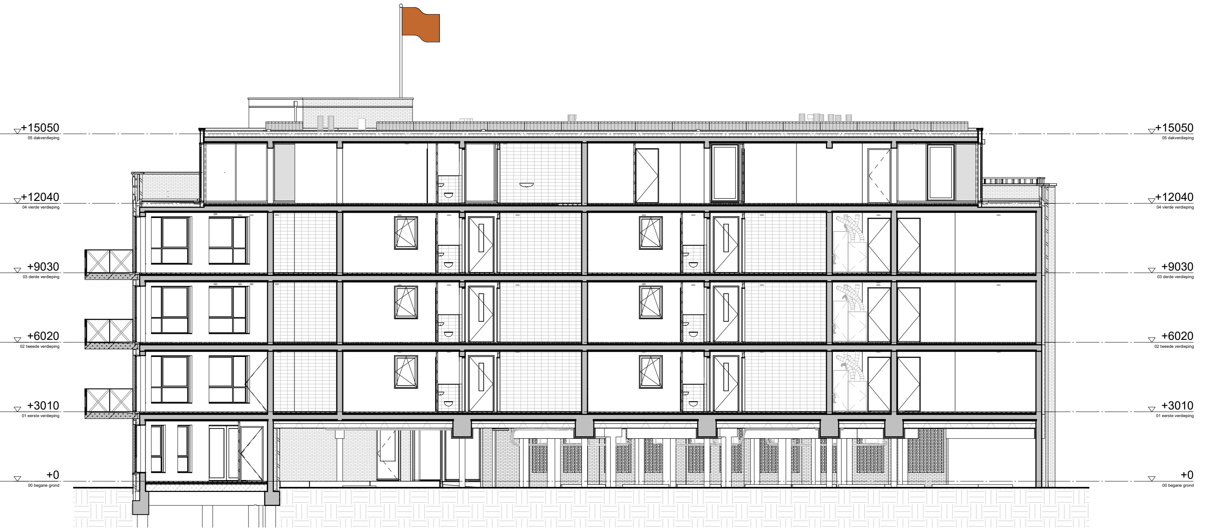
langsdoorsnede B-B Oude Vissershaven
